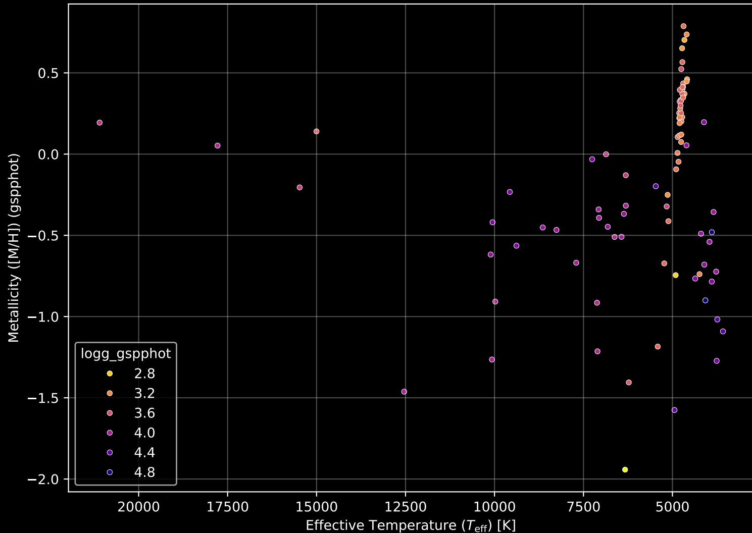
APOGEE DR17 Field: [030+00_btx] Stellar Population Parameters (n= 87)
